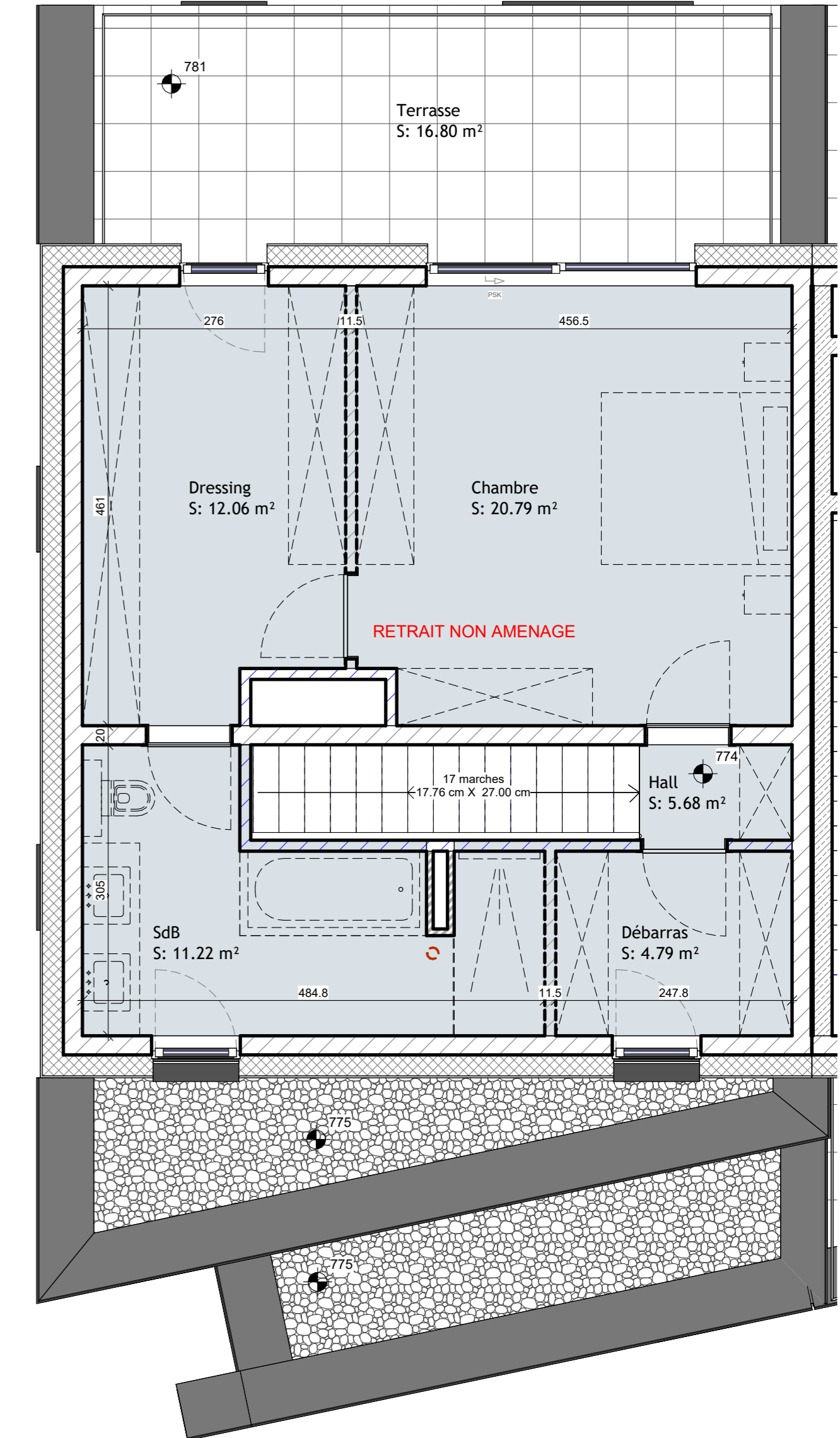
Etage 2
